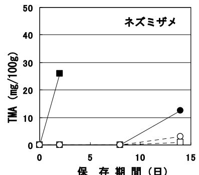
図2 保存中のサメ肉の TMA と NH 3 の変化
