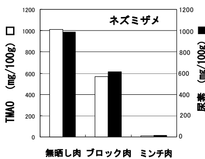
図1 水晒しによる TMAO と尿素量
